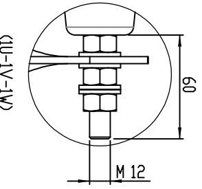
Détail A / Detail A BORNES HT / HV TERMINALS
